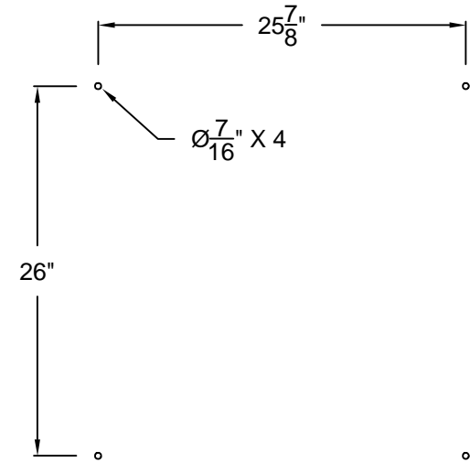
Hole Template
